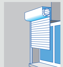
Coffre Quart de rond sur façade
